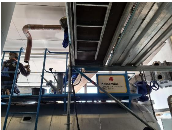
Montagearbeiten Kesselrücklauf
